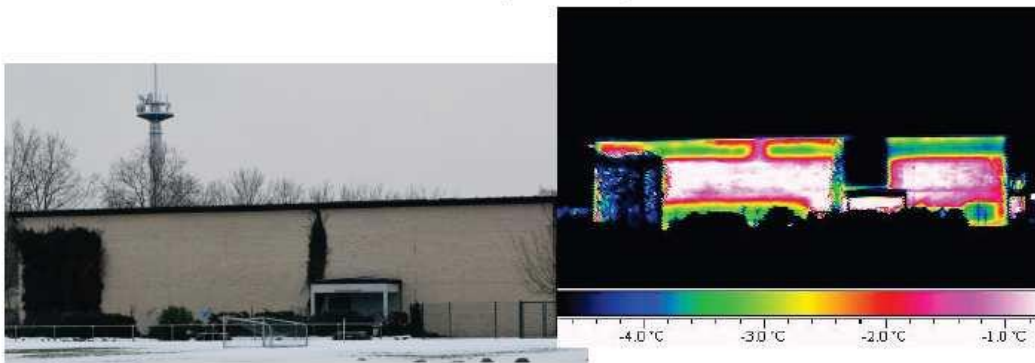
Thermogramm einer Sporthalle
